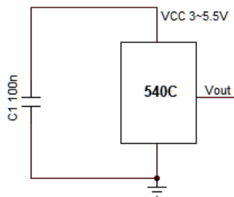
图 7 典型电路 1
