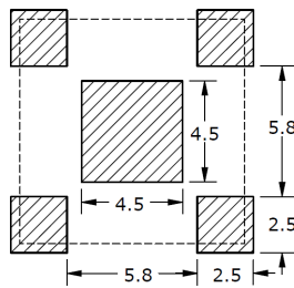
图 14 推荐焊盘
